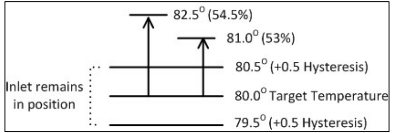
الشكل 21: مثال على تخلفية فتح فتحة التهوية
