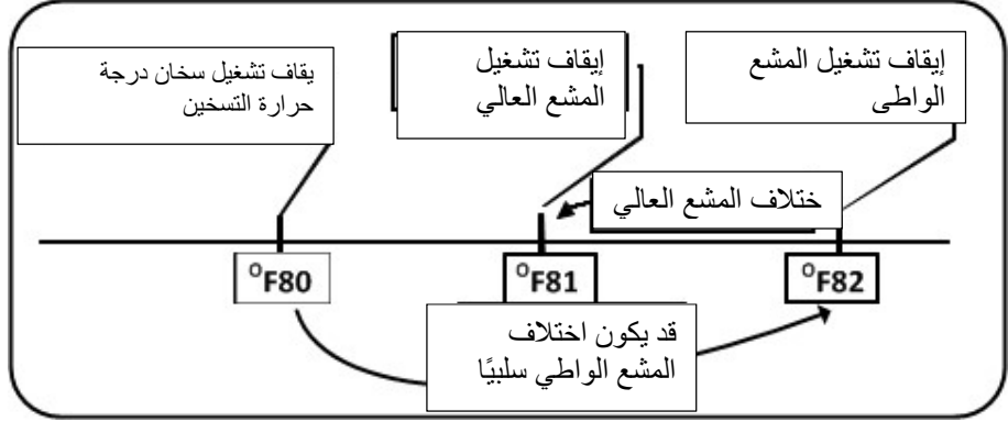
الشكل 1: اختلافات المشع الحراري
