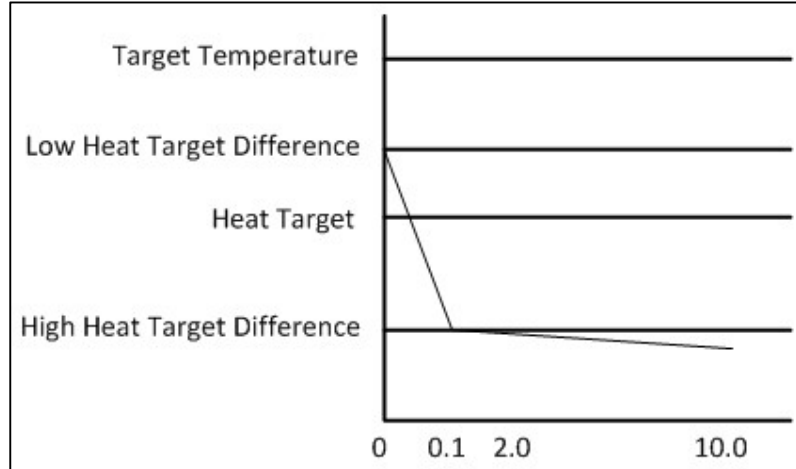
الشكل 3: مثال على السخان التناسبي
