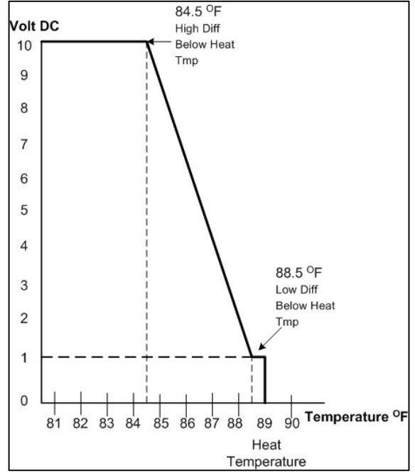
الشكل 2: مثال على سخان المتغير
