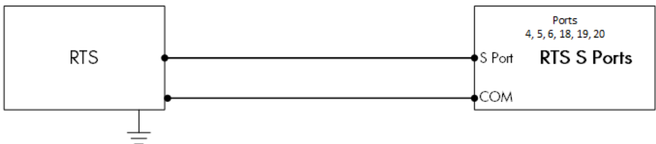
Bild 18: RTS- kopplingschema S-Port
