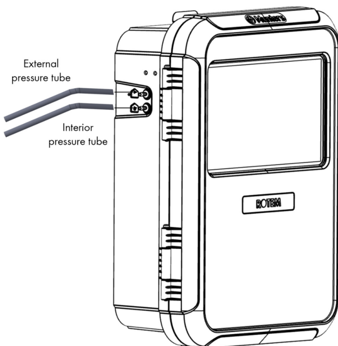
Bild 28: Slangar för statiskt tryck
