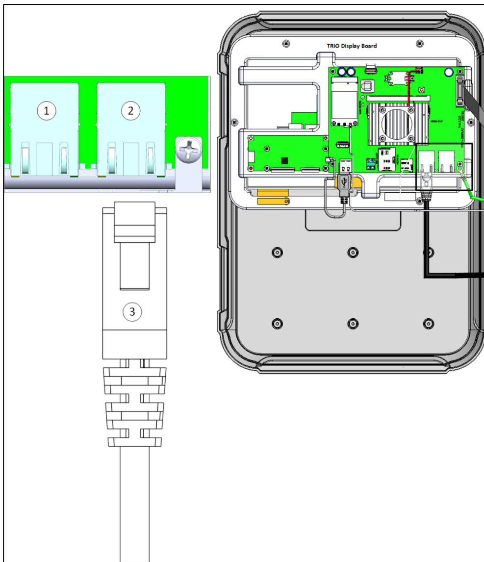
Bild 8: Ethernet-port
