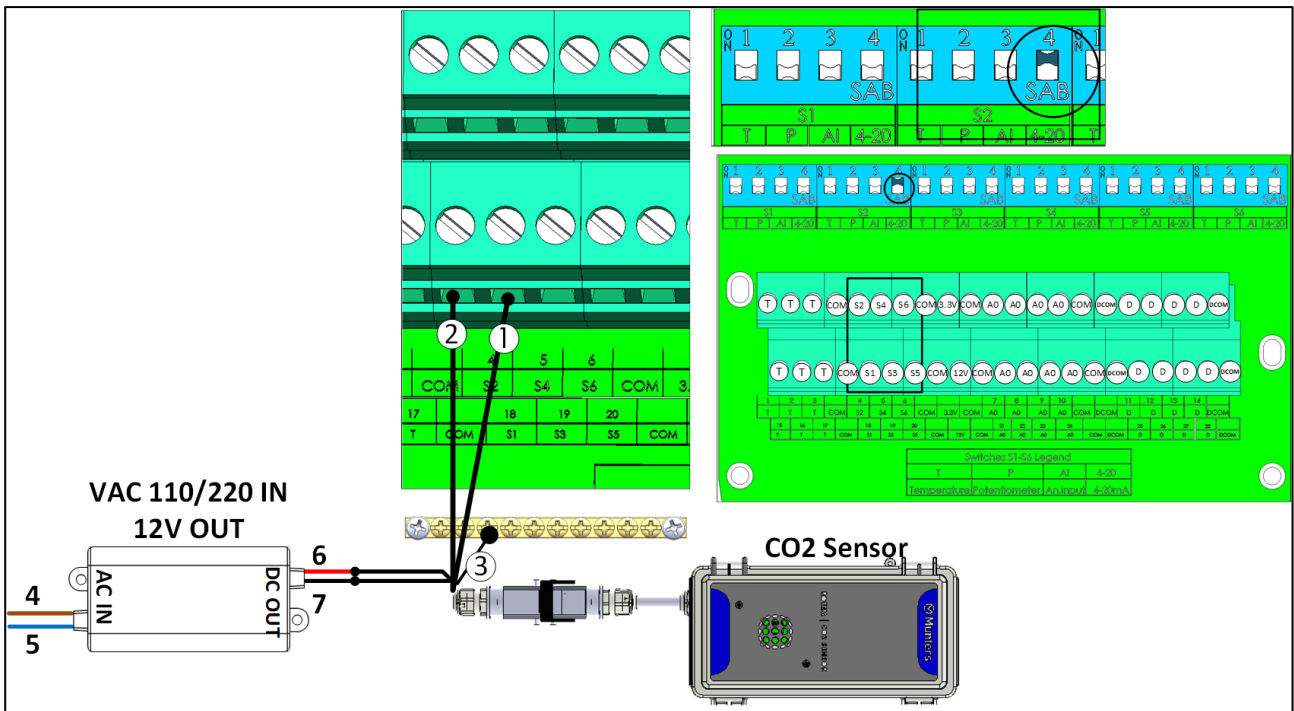
Bild 13: Ledningar för CO2-givare
