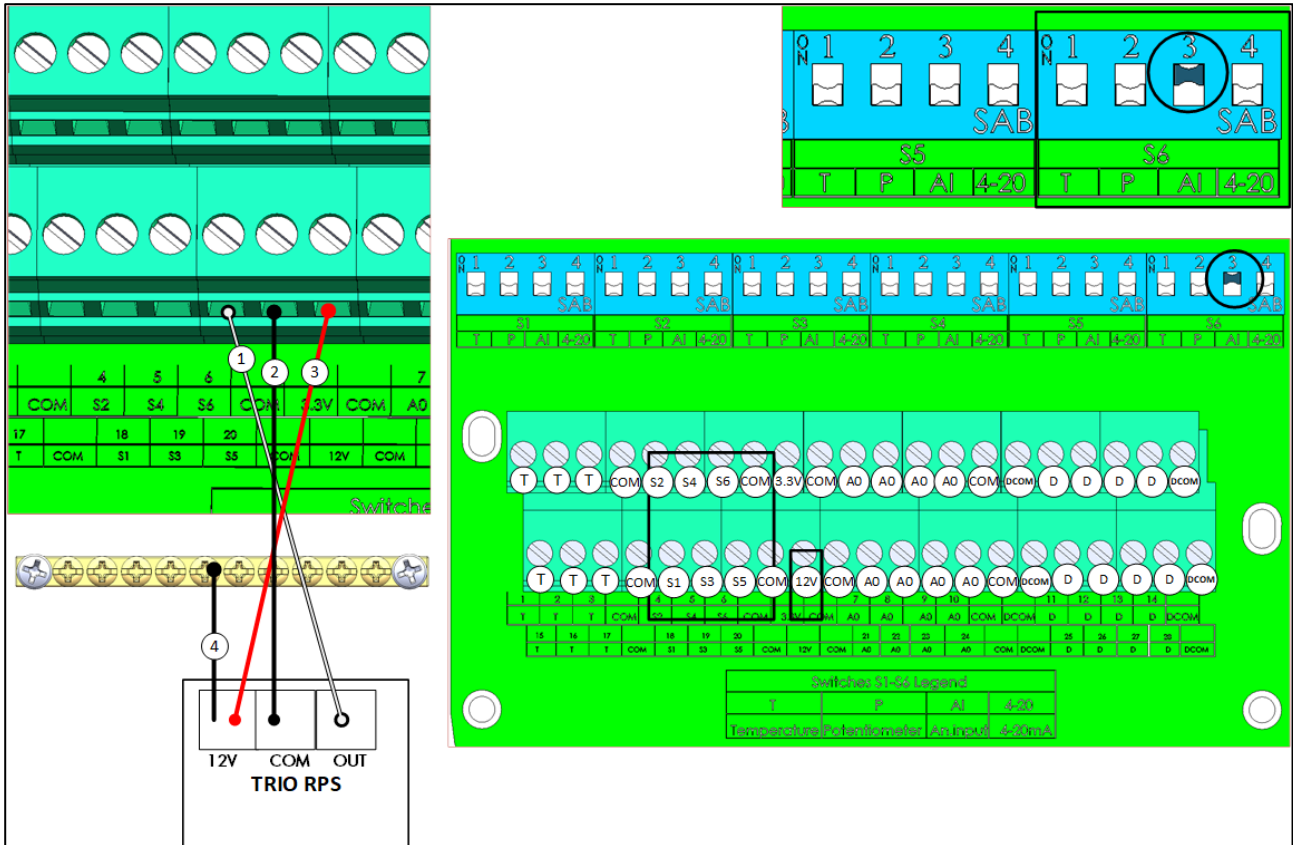
Bild 25: RPS ledning
