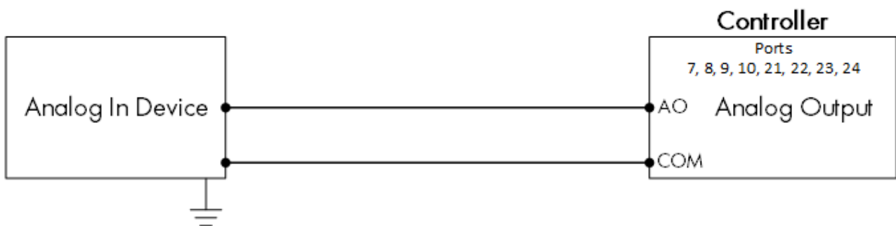
Bild 10: Schematisk kopplingschema för analoga enheter
