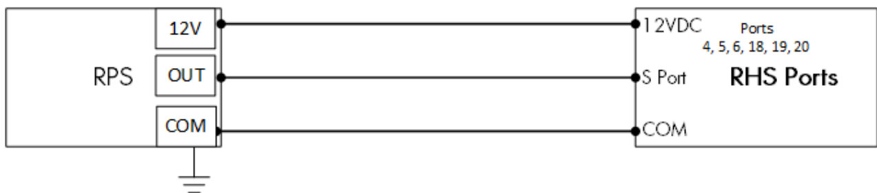
Bild 26: RPS kopplingschema
