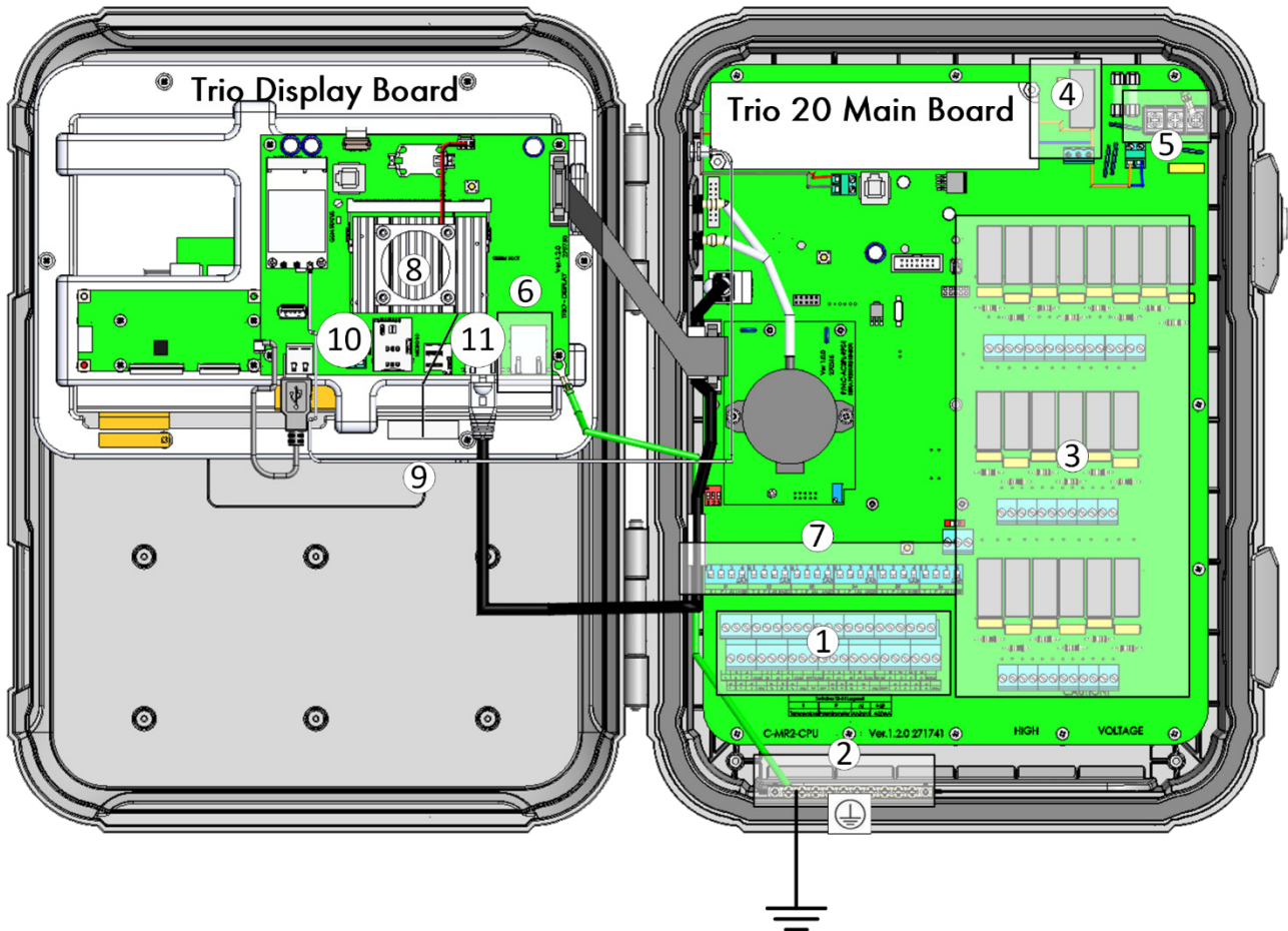
Bild 2: Layout på tavlan
