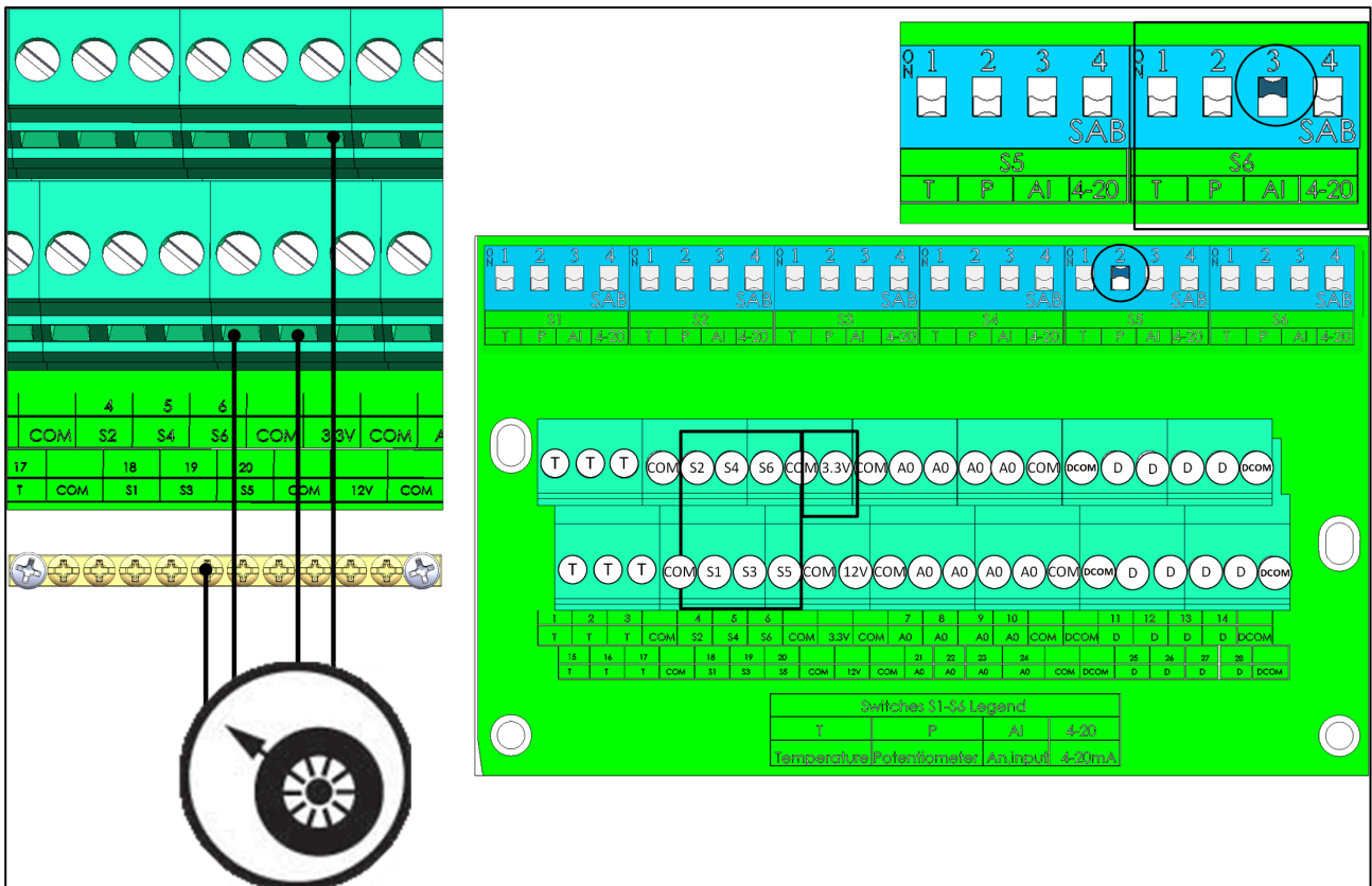
Bild 21: Potentiometers ledning
