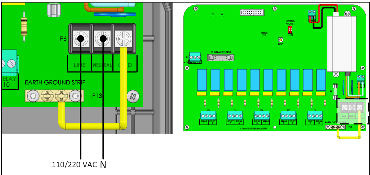
Bild 34: Strömförsörjningsportar
