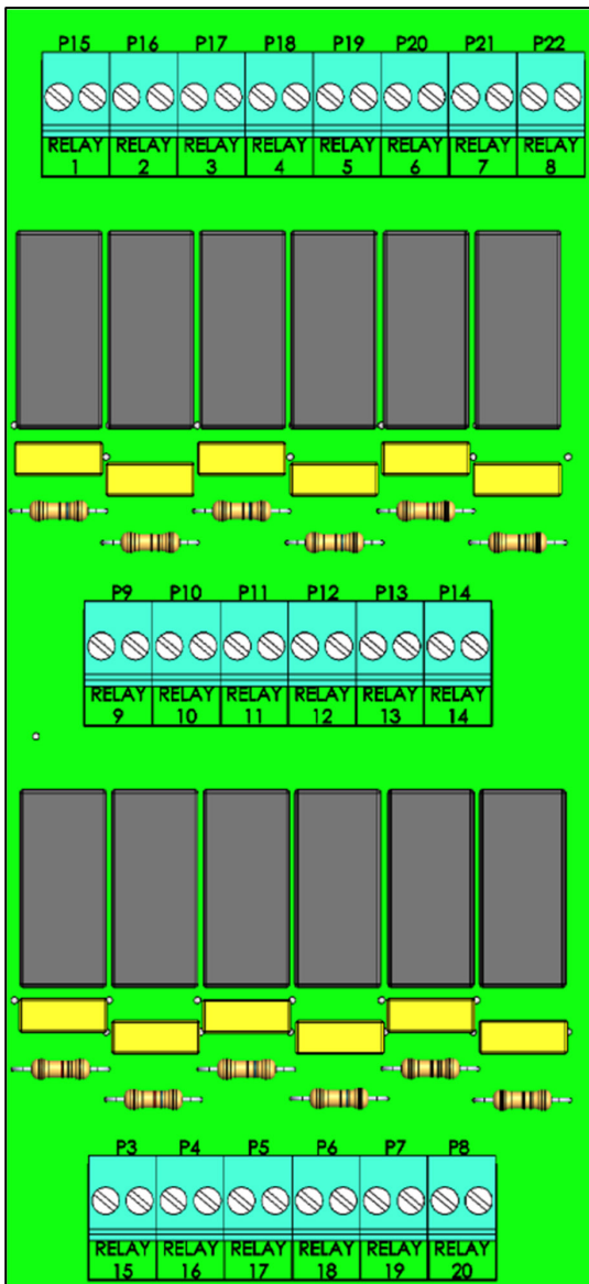
Bild 6: Relä och portnumrering
