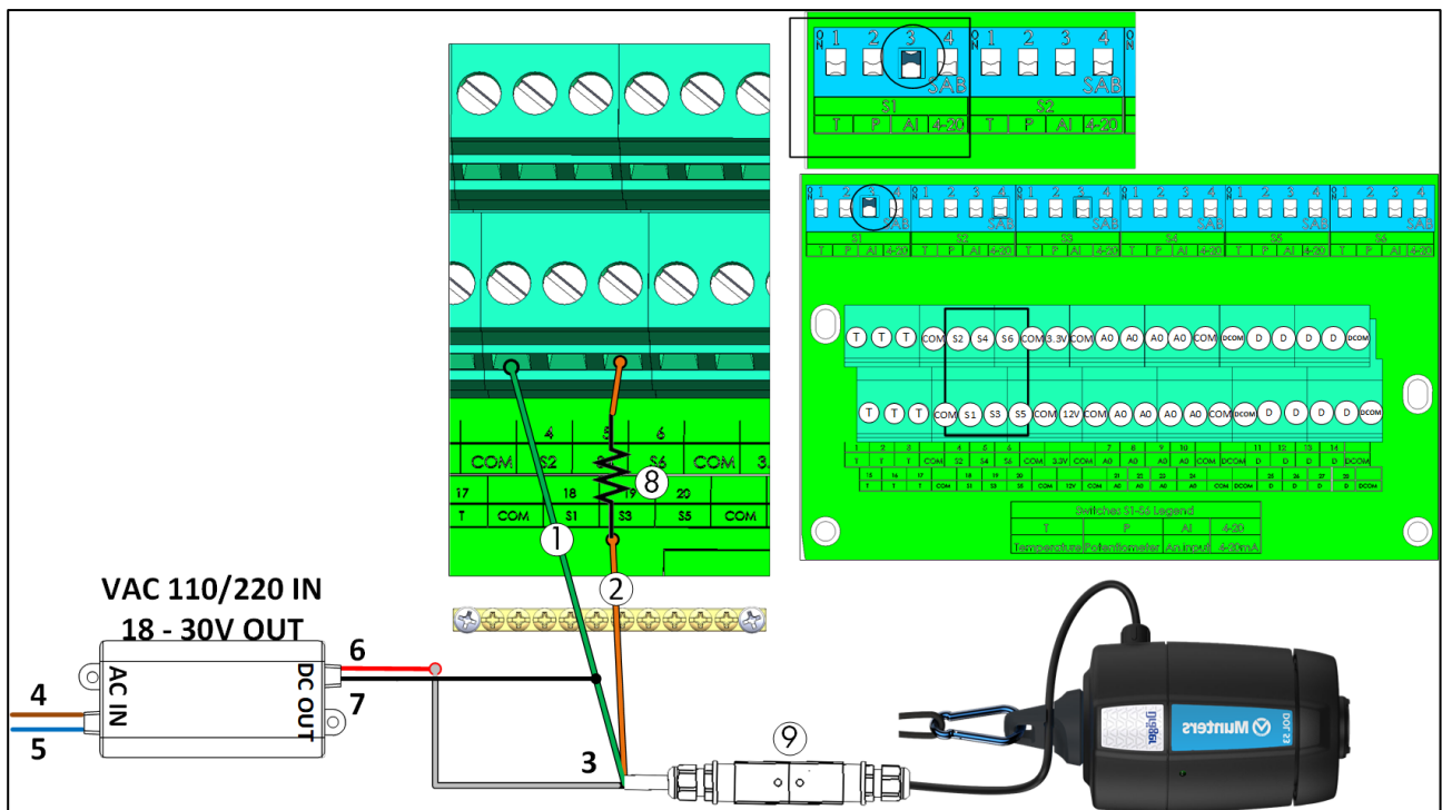
Bild 23: Ledningar för ammoniavgivare
