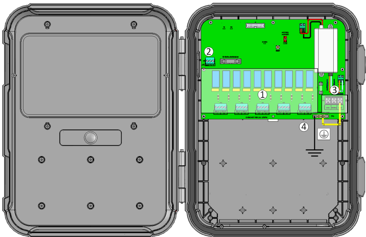
Bild 30: Layout på tavlan
