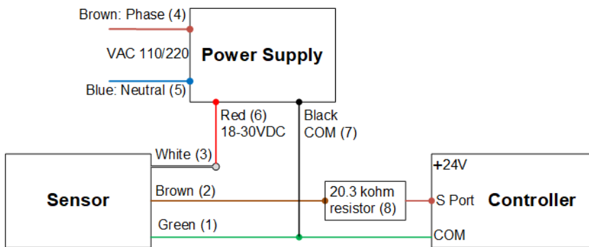
Bild 24: Ammoniak ledningsschema
