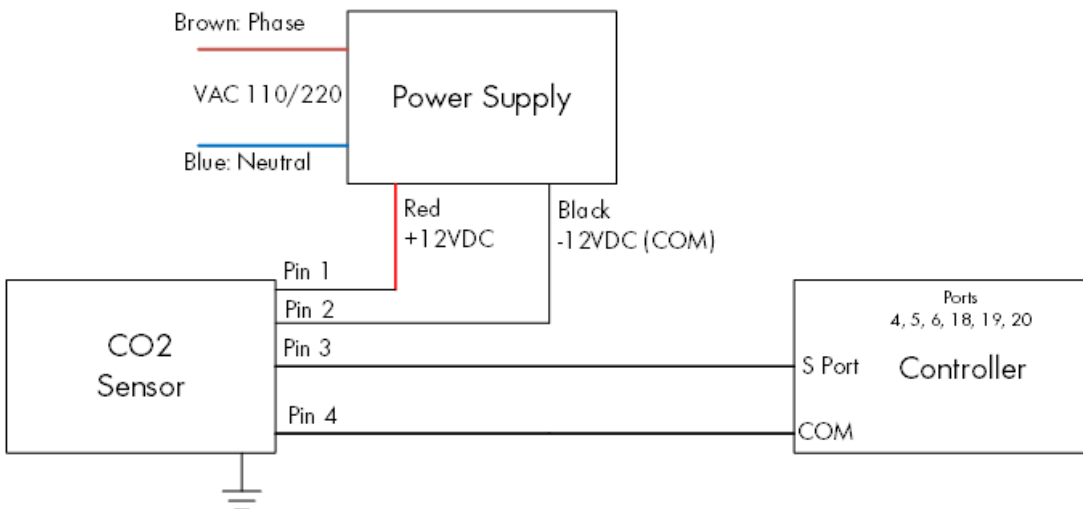
Bild 14: Schematisk kopplingschema för CO2-givare
