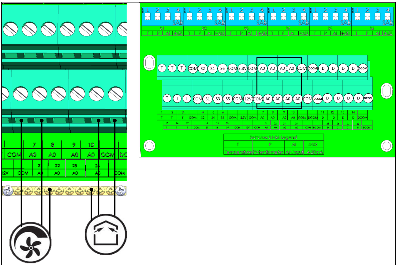
Bild 9: Analog enheter för ut-effekt(exempel)
